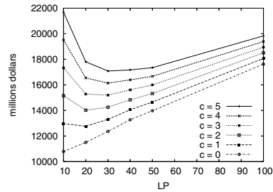
(d) Q: exp. - selection costs
